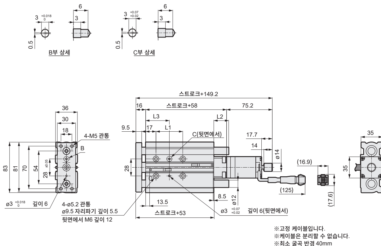
[스트로크별 치수표]
