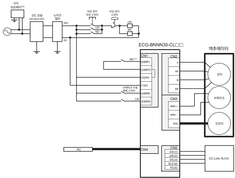
[CC-Link 타입]
